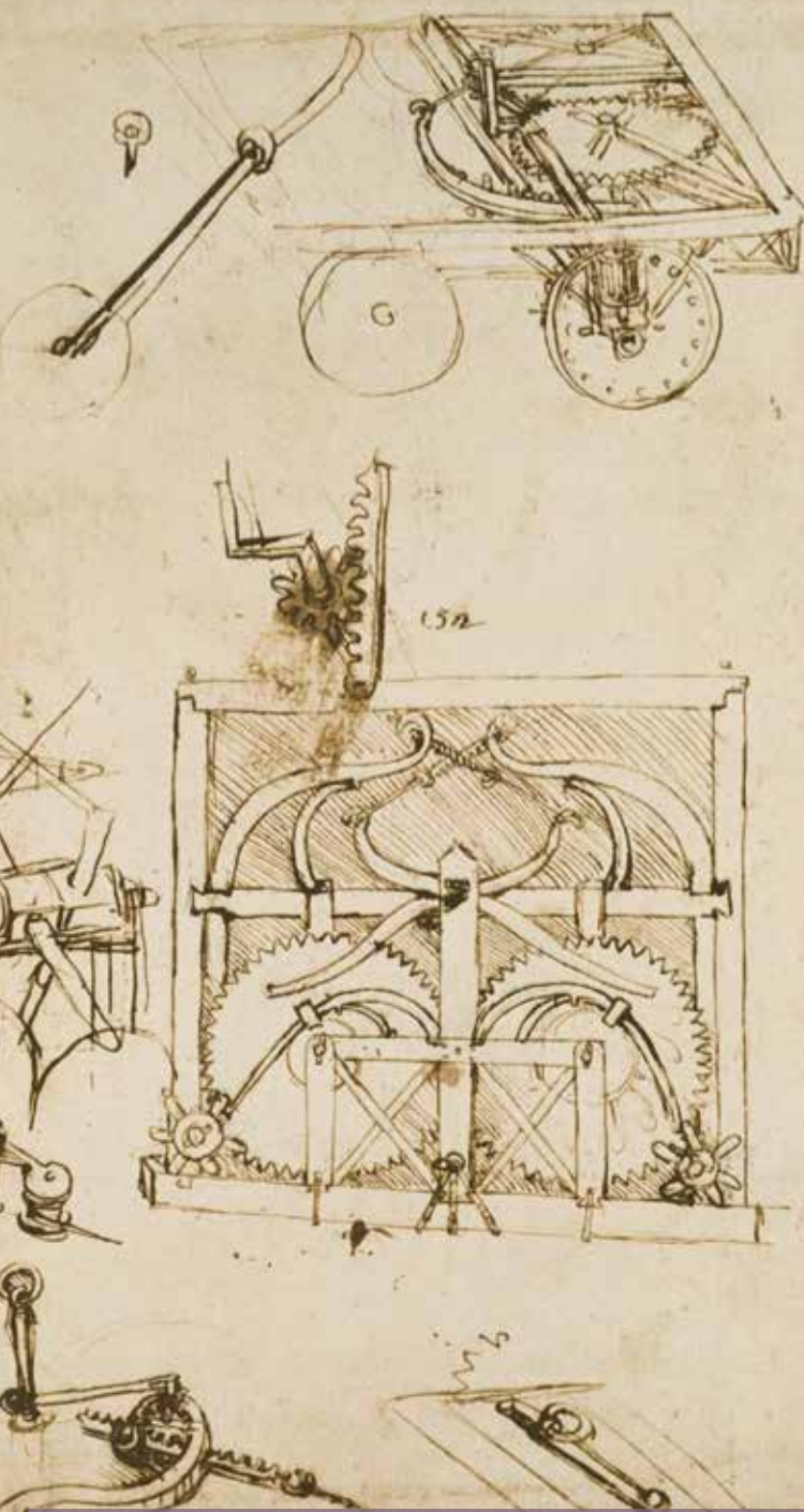
Zeichnung eines selbstfahrenden Wagens von Leonardo, um 1493
